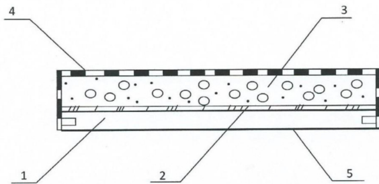
1 - konstrukcja drewniana siedziska; 2 - płyta pilśniowa; 3 - pianka poliuretanowa grubość 80 mm; 4 - tkanina dekoracyjna; 5 - podbitka (tkanina pyłochłonna).
