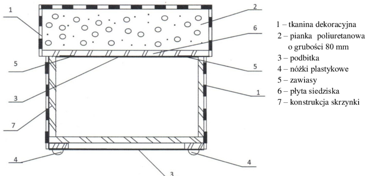
Rysunek 1. Warstwy tapicerskie pufu
