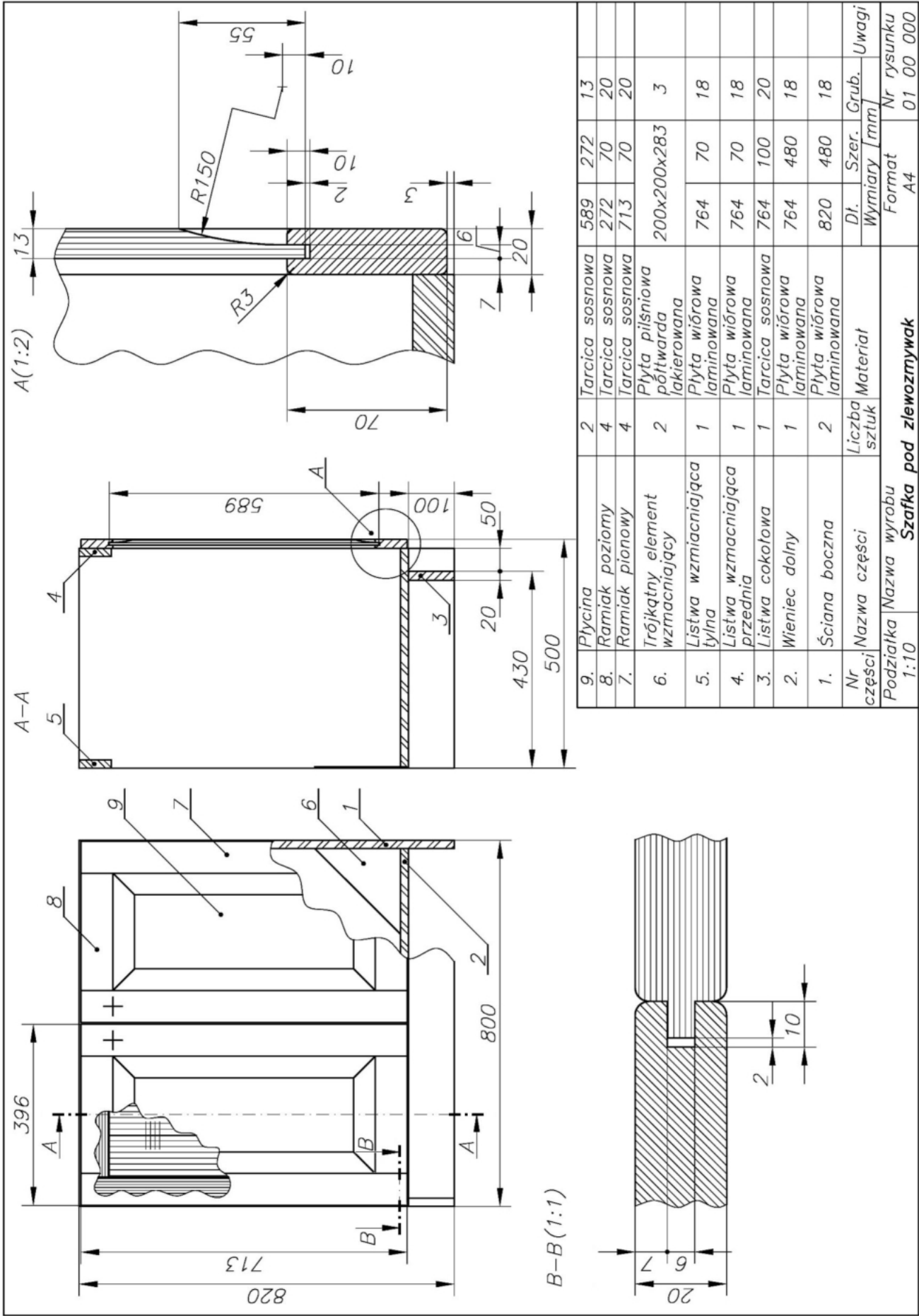
RYSUNEK ZŁOŻENIOWY SZAFKI POD ZLEWOZMYWAK
