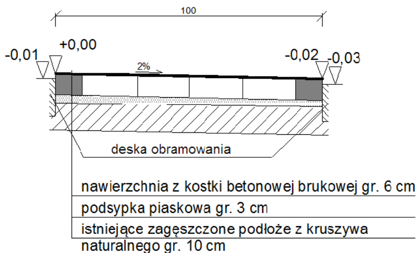
Rysunek 2. Przekrój poprzeczny nawierzchni z betonowej kostki brukowej
