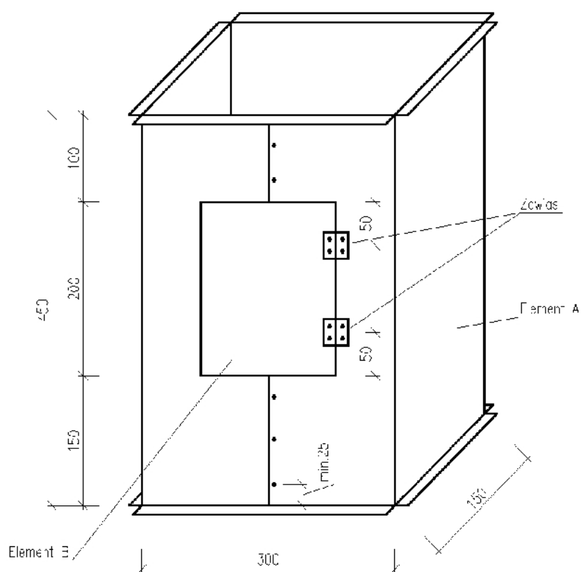
Rysunek 3. Widok kanału z zamontowaną klapą rewizyjną
