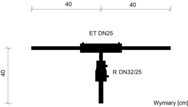
Rysunek. Fragment gazociągu PE 100 SDR 11 DN 32 i DN 25
