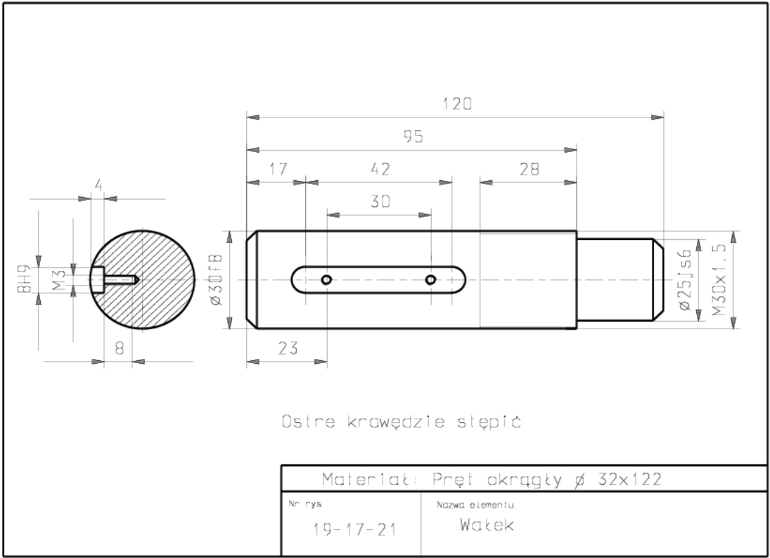
Rysunek 19-17-21 Wałek
