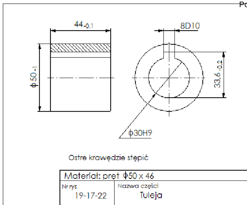
Rysunek 19-17-22 Tuleja
