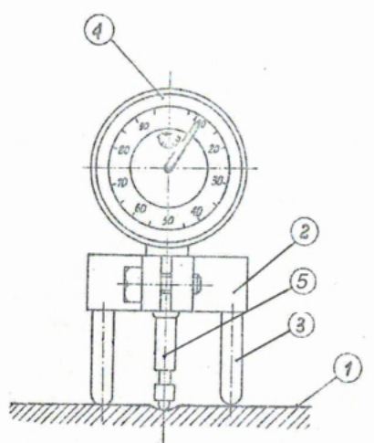
Rys. 1. Pomiar głębokości wgnieceń
